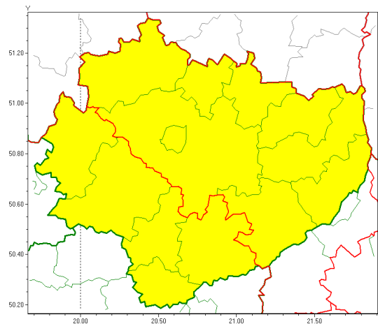
Burze z gradem 2019-08-28 12:41
