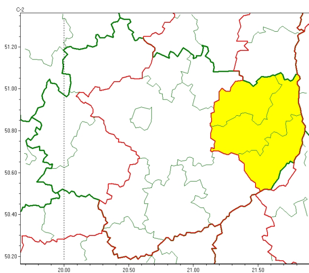
Opady marznące 2023-04-06 10:34
